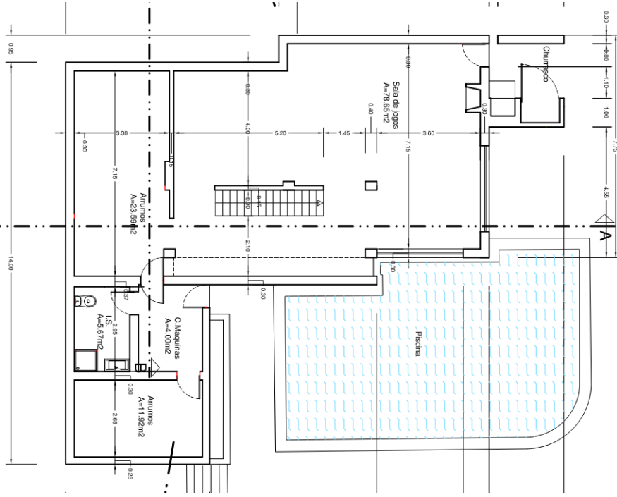
Piso 0
