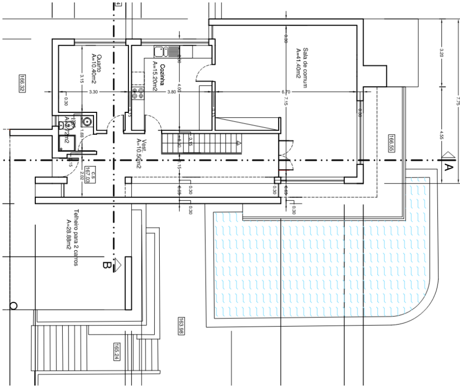
Piso 1
